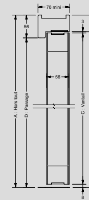
Coupe horizontale 2 vantaux (joint double lèvres)
