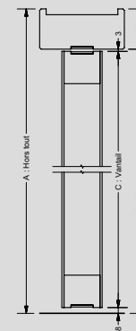
Coupe verticale
