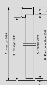
Coupe verticale
