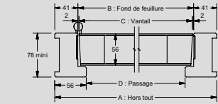
Coupe horizontale 1 vantail
