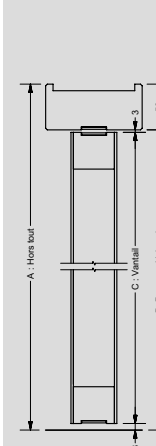
Coupe verticale
