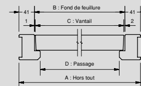
Coupe horizontale 1 vantail
