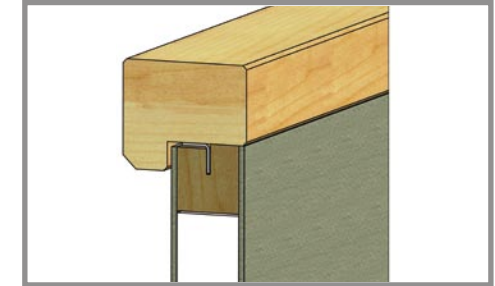
Cornière posée sur traverse d'imposte.
