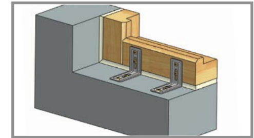
Pose du bloc-porte avec équerre (non fournie).
