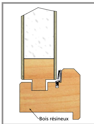
Trappe d'accès aux combles isolante. Rainurage pour une fixation optimale.
