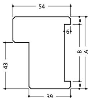
Huisserie
