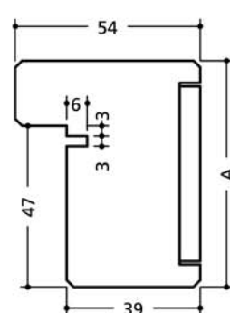
Bâti option joint d'étanchéité
