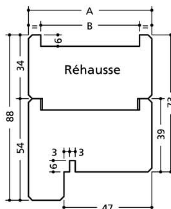
Huisserie option joint d'étanchéité
