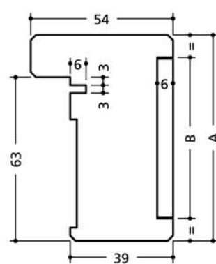
Bâti option joint d'étanchéité
