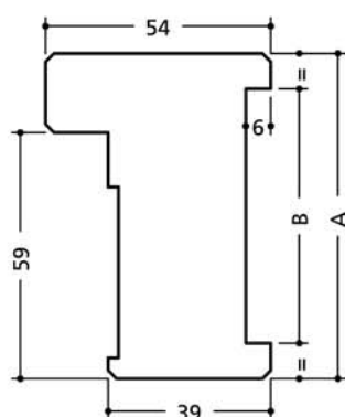
Huisserie
