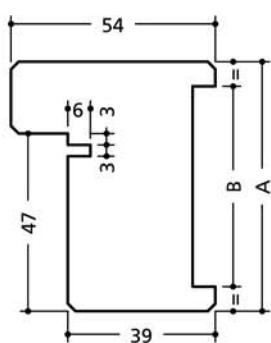
Huisserie option joint d'étanchéité
