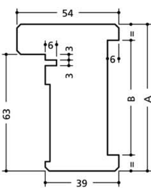
Huisserie option joint d'étanchéité
