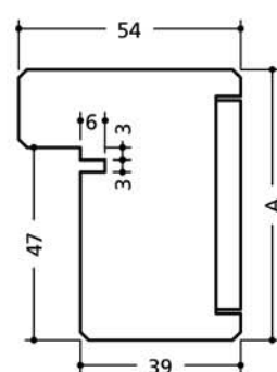
Bâti option joint d'étanchéité
