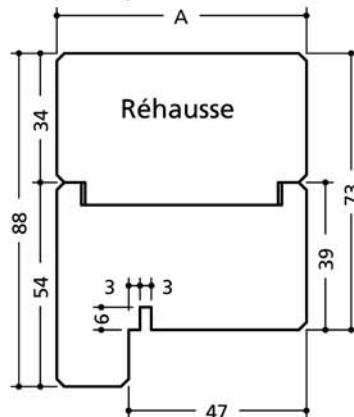
Bâti option joint d'étanchéité
