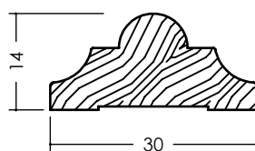
Profil 30x14
