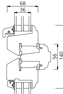
TRANSOM
