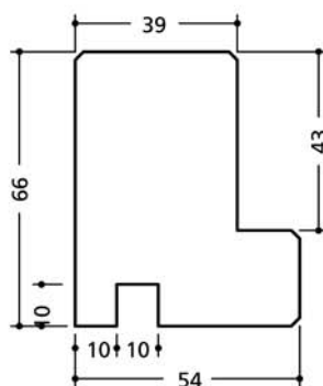
Bâti Rainure côté cochonnet
