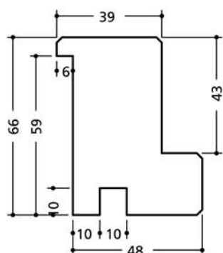
Type A1 + Rainure ébrasement
