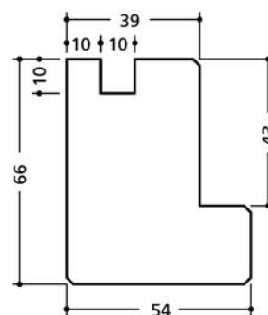
Bâti Rainure côté paumelles
