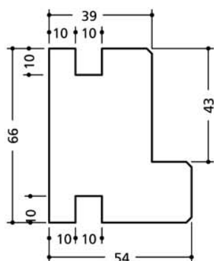
Bâti 2 rainures
