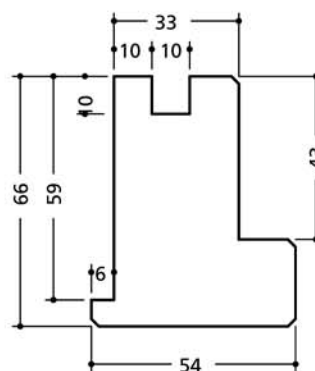
Type A2 + Rainure ébrasement
