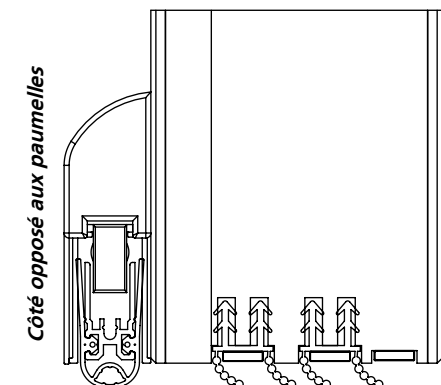
Double Joints Balais + Plinthe Applique
