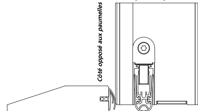
Plinthe Encastrée + Seuil
