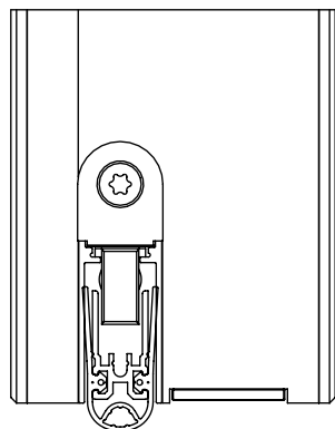
Plinthe Encastrée
