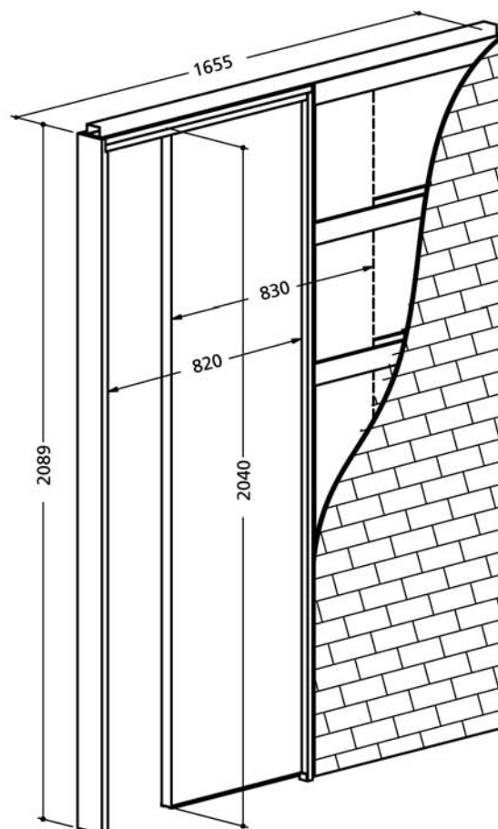
Type 6 - Cuvette + trou de doigt + mortaise têteière pour serrure à crochet à cylindre
