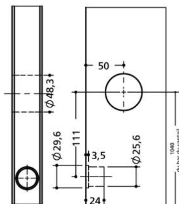
Type 2 Cuvette + trou de doigt
