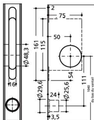
Type 6 - Cuvette + trou de doigt + mortaise têteière pour serrure à crochet à cylindre
