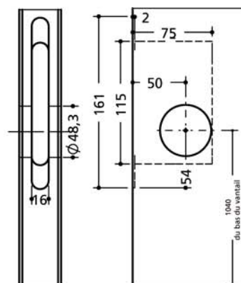
Type 6 - Cuvette + trou de doigt + mortaise têteière pour serrure à crochet à cylindre
