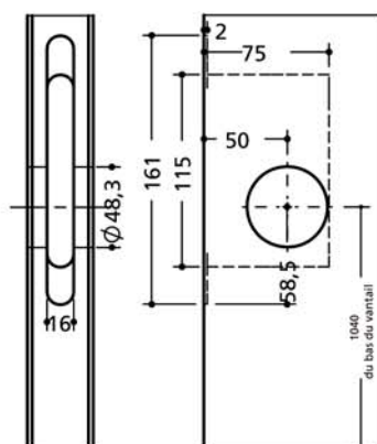
Type 5 - Cuvette + trou de doigt + mortaise têteière pour serrure à crochet BCC ou PDDT
