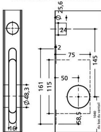
Type 5 - Cuvette + trou de doigt + mortaise têteière pour serrure à crochet BCC ou PDDT
