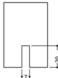
Détail rainure basse
