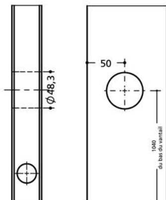
Type 1 Cuvette seule
