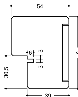
Bâti avec joint d'étanchéité
