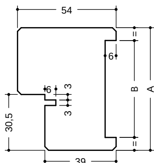
Huisserie avec joint d'étanchéité
