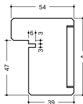
Bâti avec joint d'étanchéité
