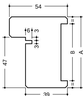
Huisserie avec joint d'étanchéité
