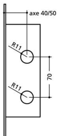
Bec de cane à condamnation
