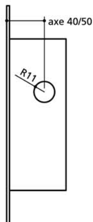
Serrure sûreté
